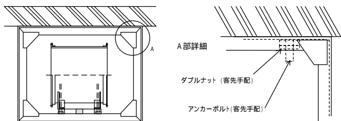
図 8 AIM型 籠形天井吊り取付(例)
