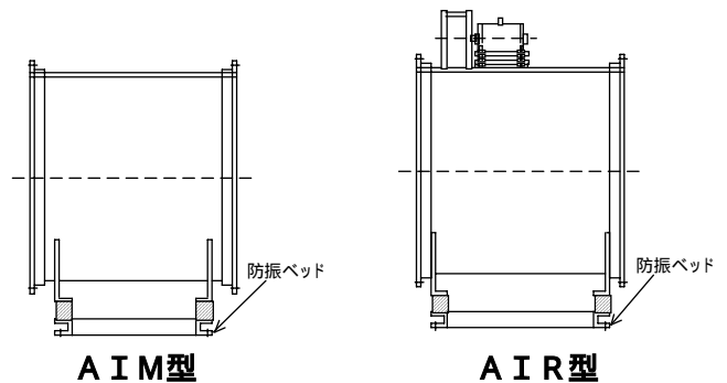
図 2 床置型（例）
