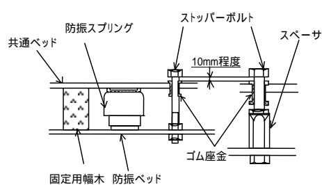
図 7 防振スプリング付の場合
