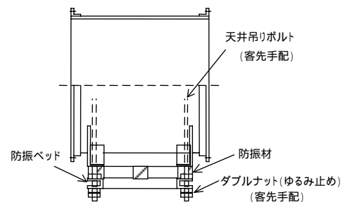
図 5 AIM型 天井吊り型防振スプリング付（例）
